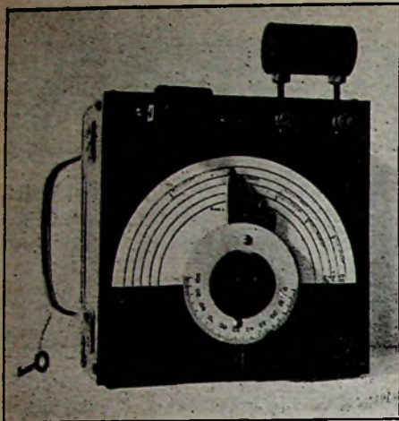
Standaardtype golfmeter van het QRH-bureau.
