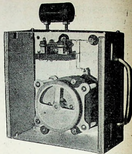
Het inwendige van den golfmeter.
