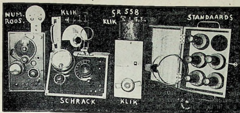
Installatie voor het ijken van golfmeters van het QRH-bureau.
